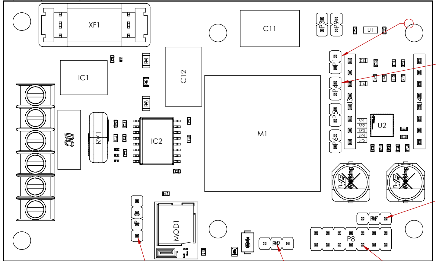
Top side (Scale 2:1)
